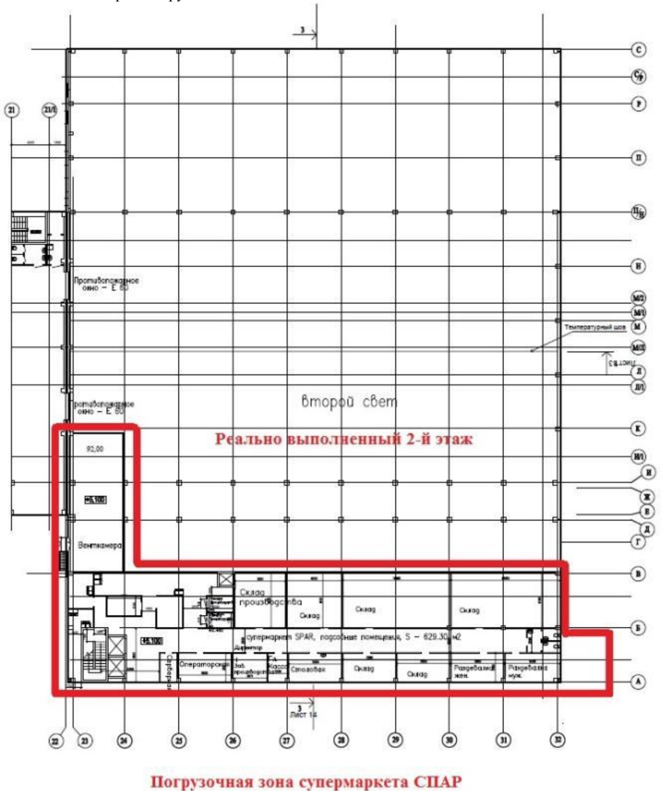
Приложение 12. Местоположение незаконно выполненного второго этажа в осях «А-В/23-32» и «А-К/23-24». 2-я реконструкция.
